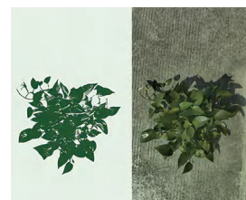
植被覆盖度
