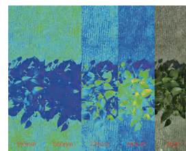
单波段渲染
