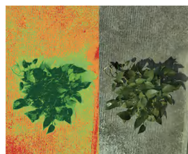
植被指数
